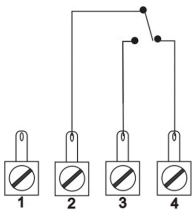
Shema spajanja PIT 92-t
